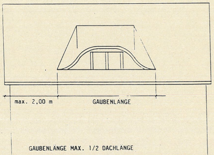
OCHSENAUGENGAUBE
