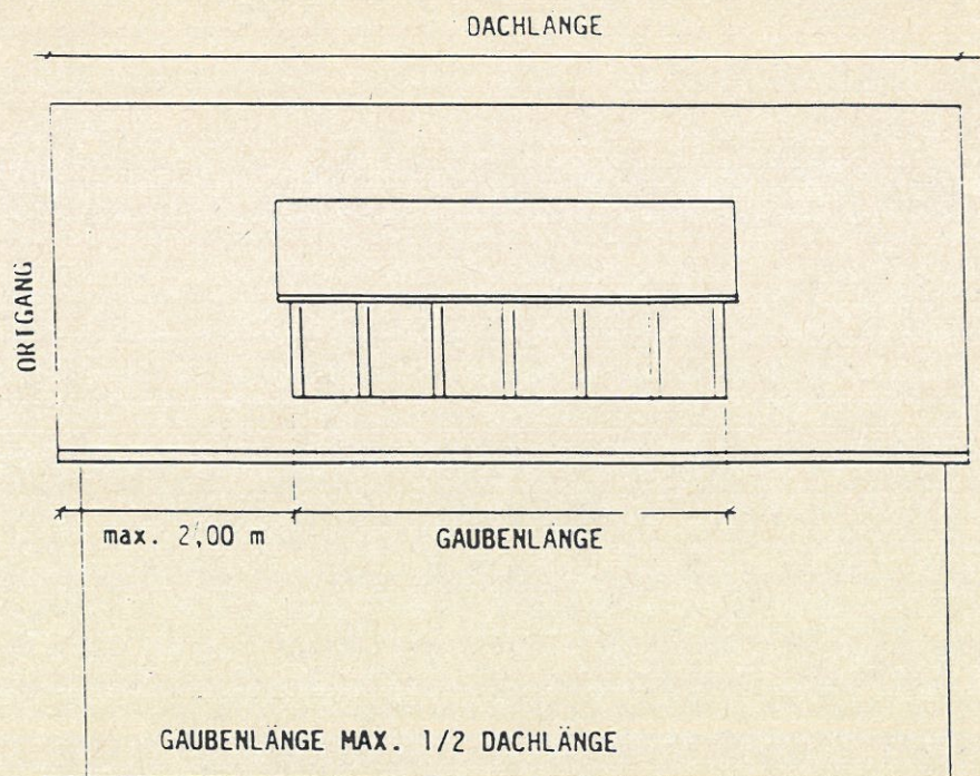
SATTELDACHGAUBE
